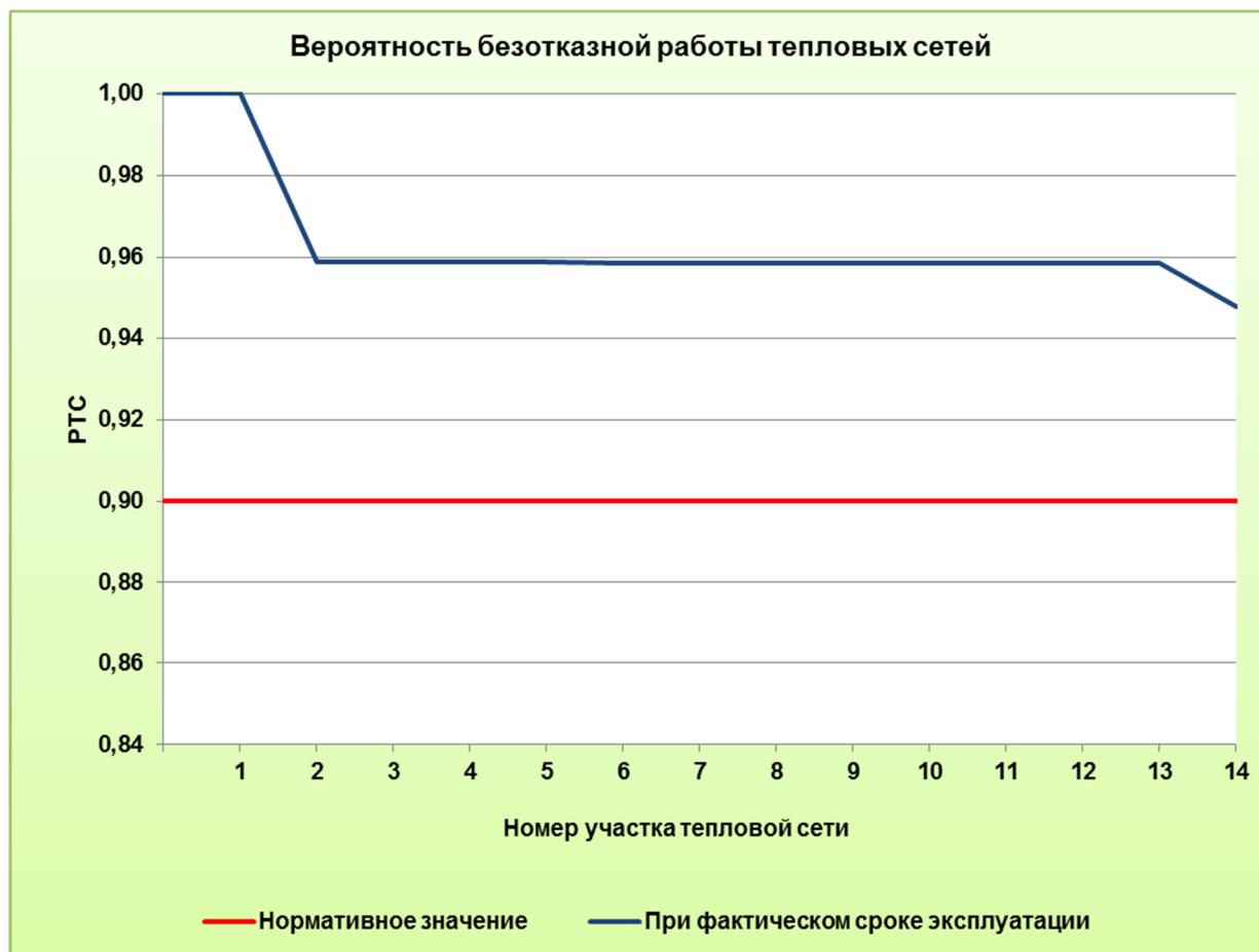
Рисунок 2.8 Вероятность безотказной работы тепловых сетей от Архангельской ТЭЦ до ТК-18т-4
