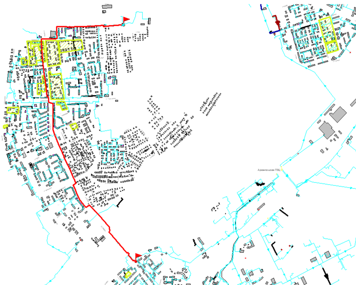
Рисунок 2.1 – Путь для расчёта вероятности безотказной работы тепловых сетей от ТК-45 до С-28п-16
