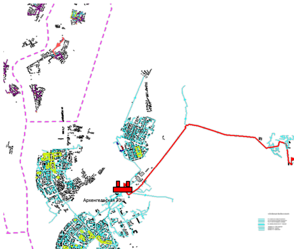
Рисунок 2.5 – Путь для расчёта вероятности безотказной работы тепловых сетей от Архангельской ТЭЦ до ТК-18т-4
